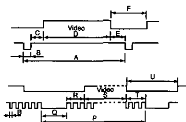
Sincronización compuesta H / V
