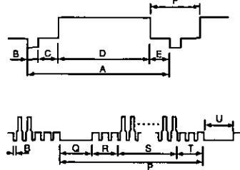
Sincronización en el verde
